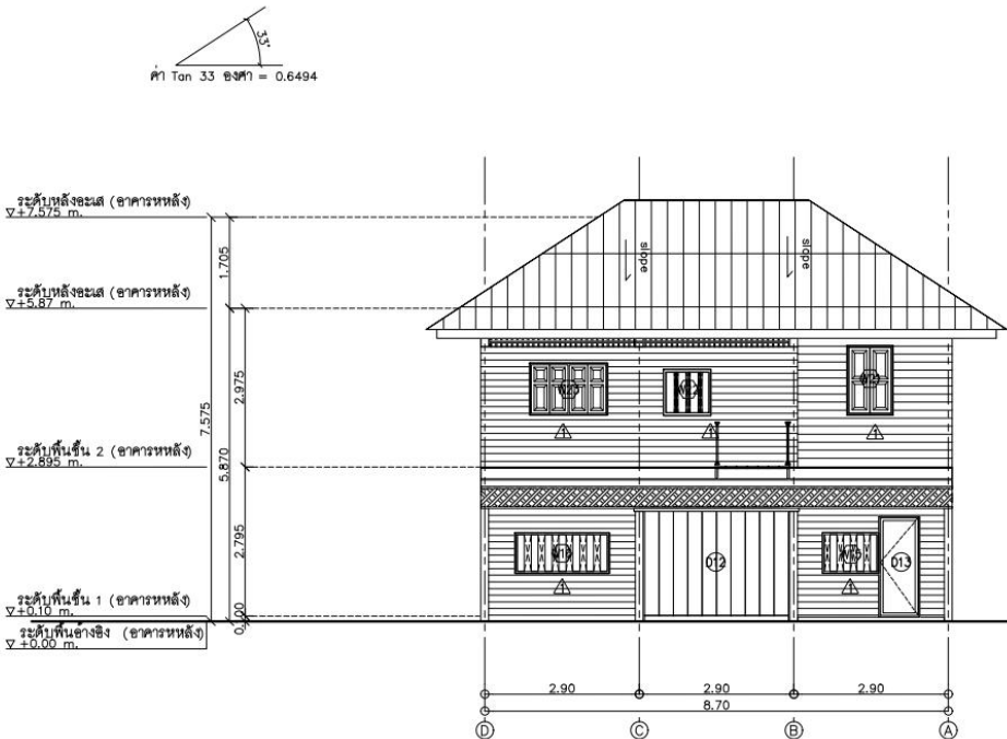
รูปด้าน A อาคารด้านหน้า
