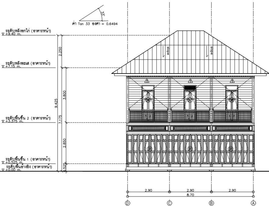
รูปด้าน A อาคารด้านหน้า มาตราส่วน 1:125
