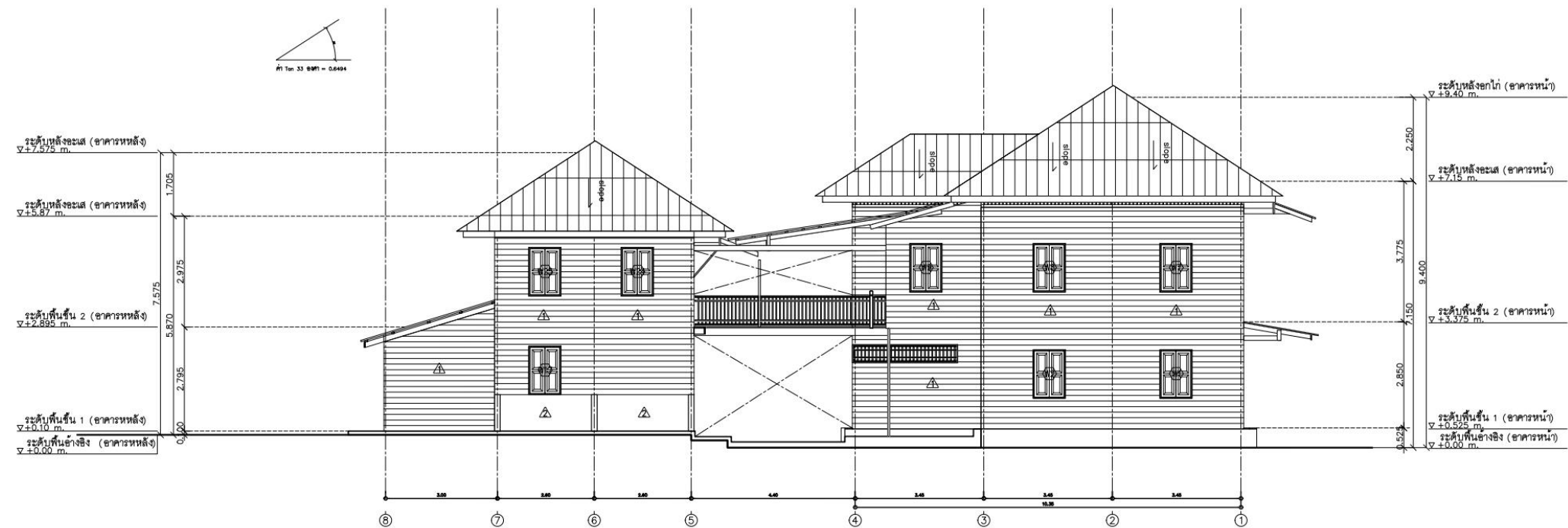
รูปด้าน B อาคารด้านหน้า ด้านหลัง และทางเชื่อม มาตราส่วน 1:125
