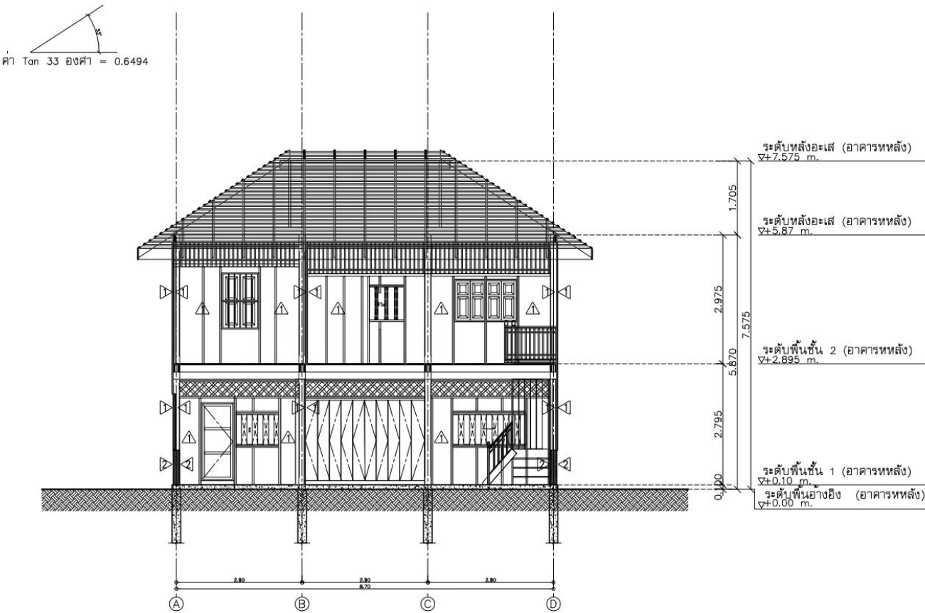
รูปตัด C อาคารด้านหลัง มาตราส่วน 1:100
