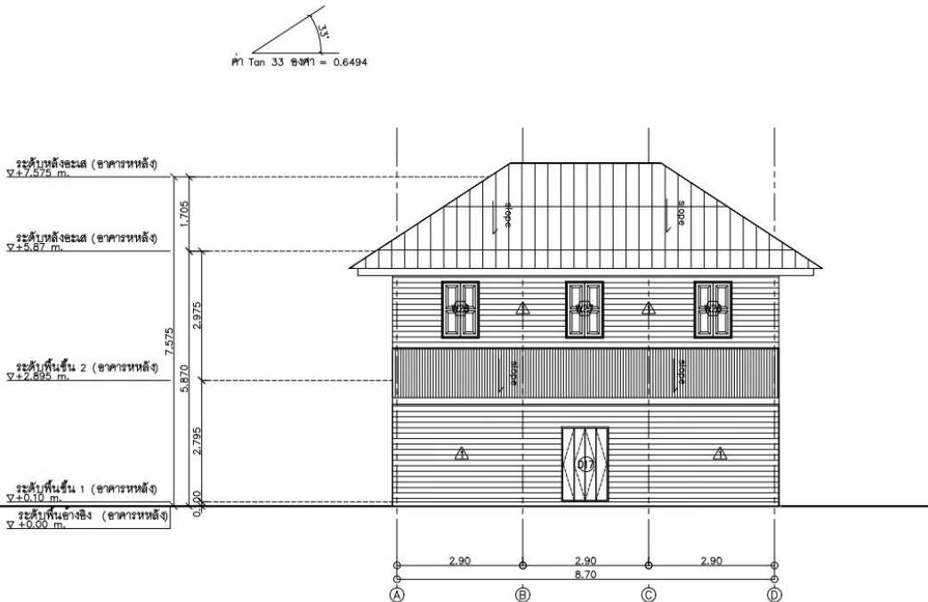
รูปด้าน C อาคารด้านหน้า
