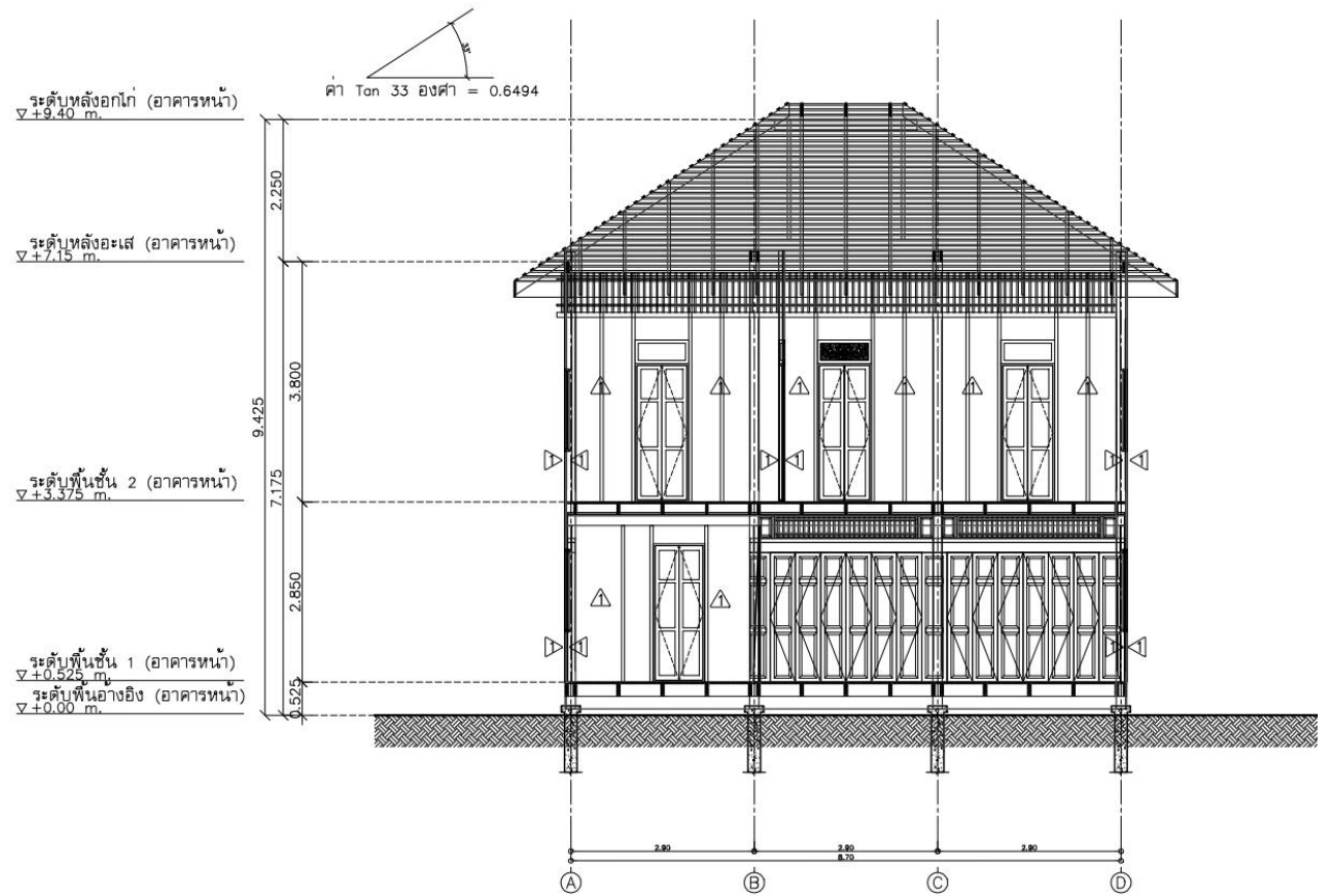
รูปตัด B อาคารด้านหน้า มาตราส่วน 1:100
